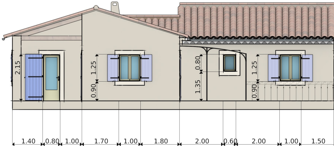
Façade Sud
